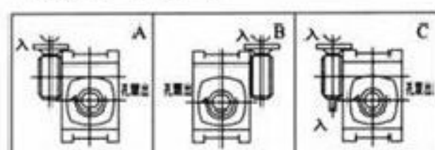
轴指向表示
