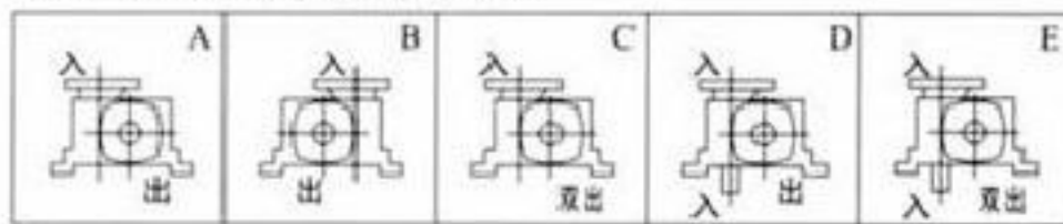
WPWDT轴指向表示
