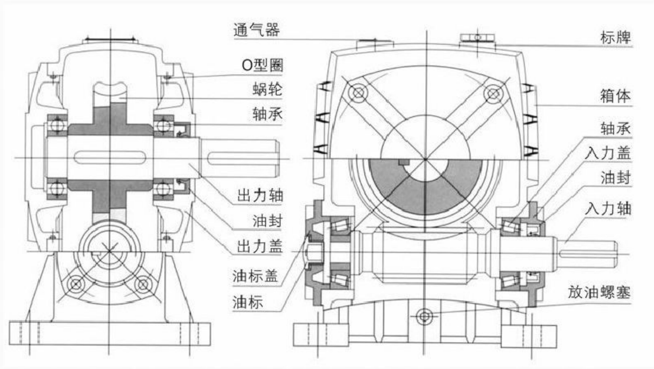
WP系列涡轮减速机产品结构图
