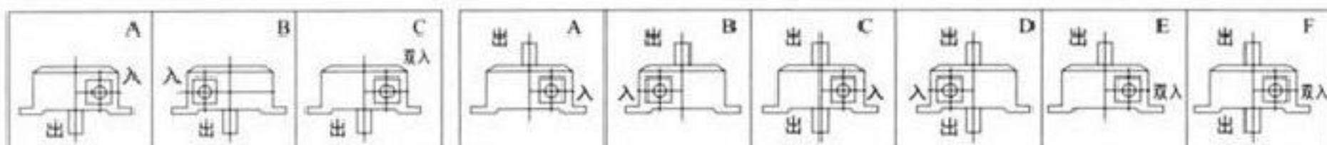
WPX轴指向表示
