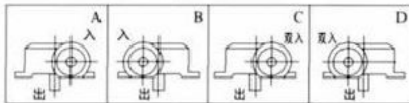
WPWDX轴指向表示
