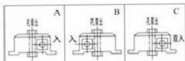
轴指向表示
