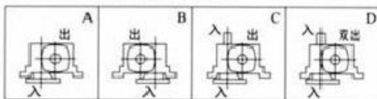
WPWDV轴指向表示
