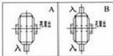
轴指向表示
