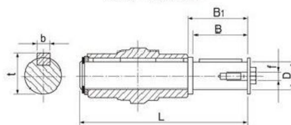
AS单向输出轴
