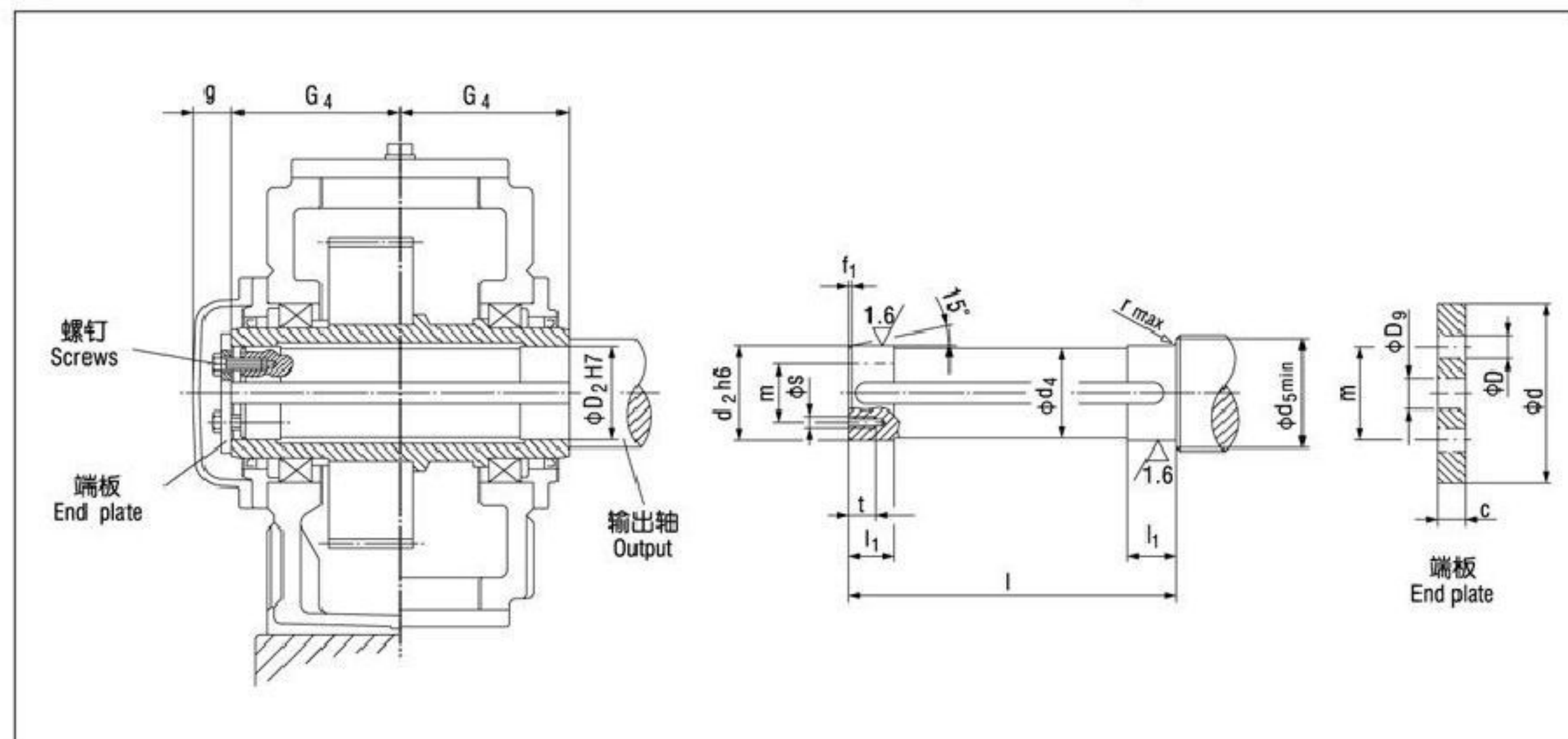
带平键联接的空心轴尺寸图表:
