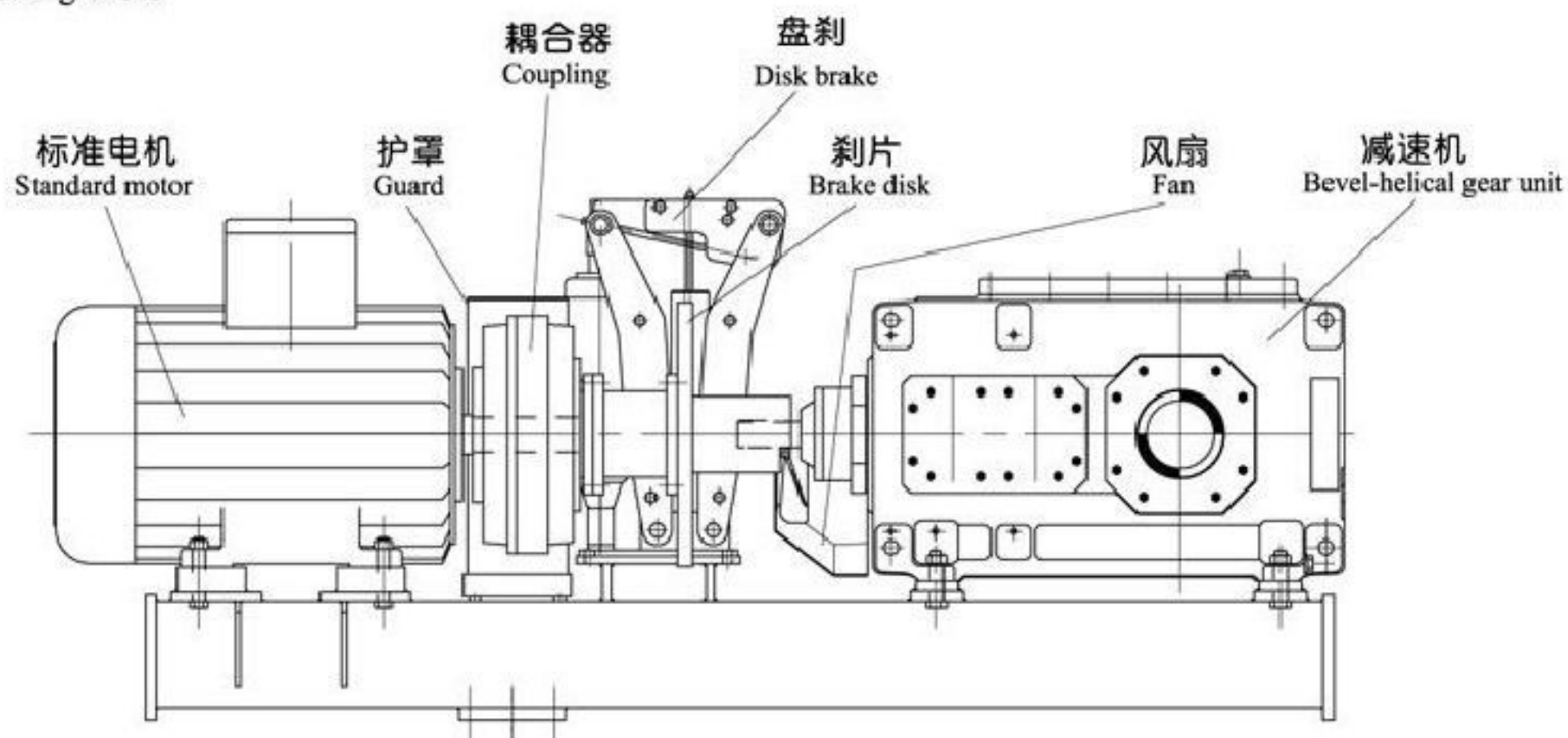
带齿轮箱摆动底座 Gear unit swing-bases
